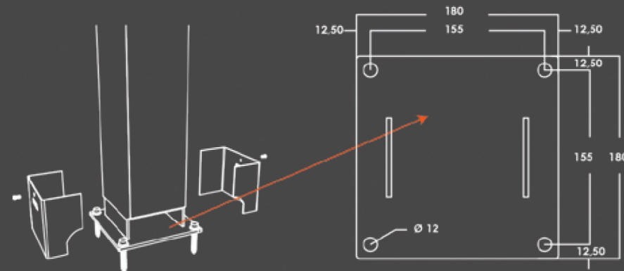
■ Βάση στήριξης κολώνας 130 x 130 Column support base 130 x 130
