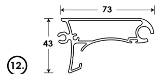
Ext. Bottom Bar
